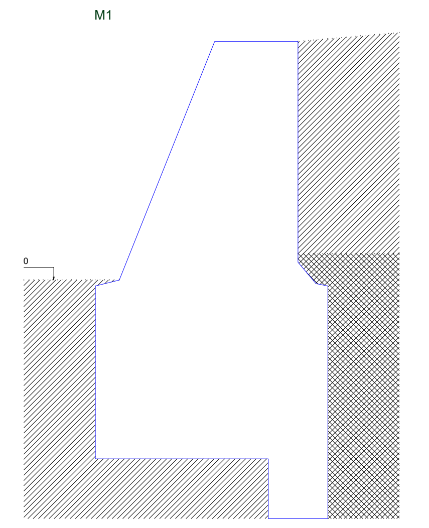
Legenda dos muros
